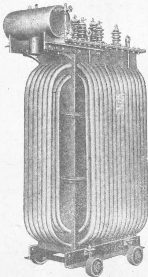
1000 KVA 變壓器
